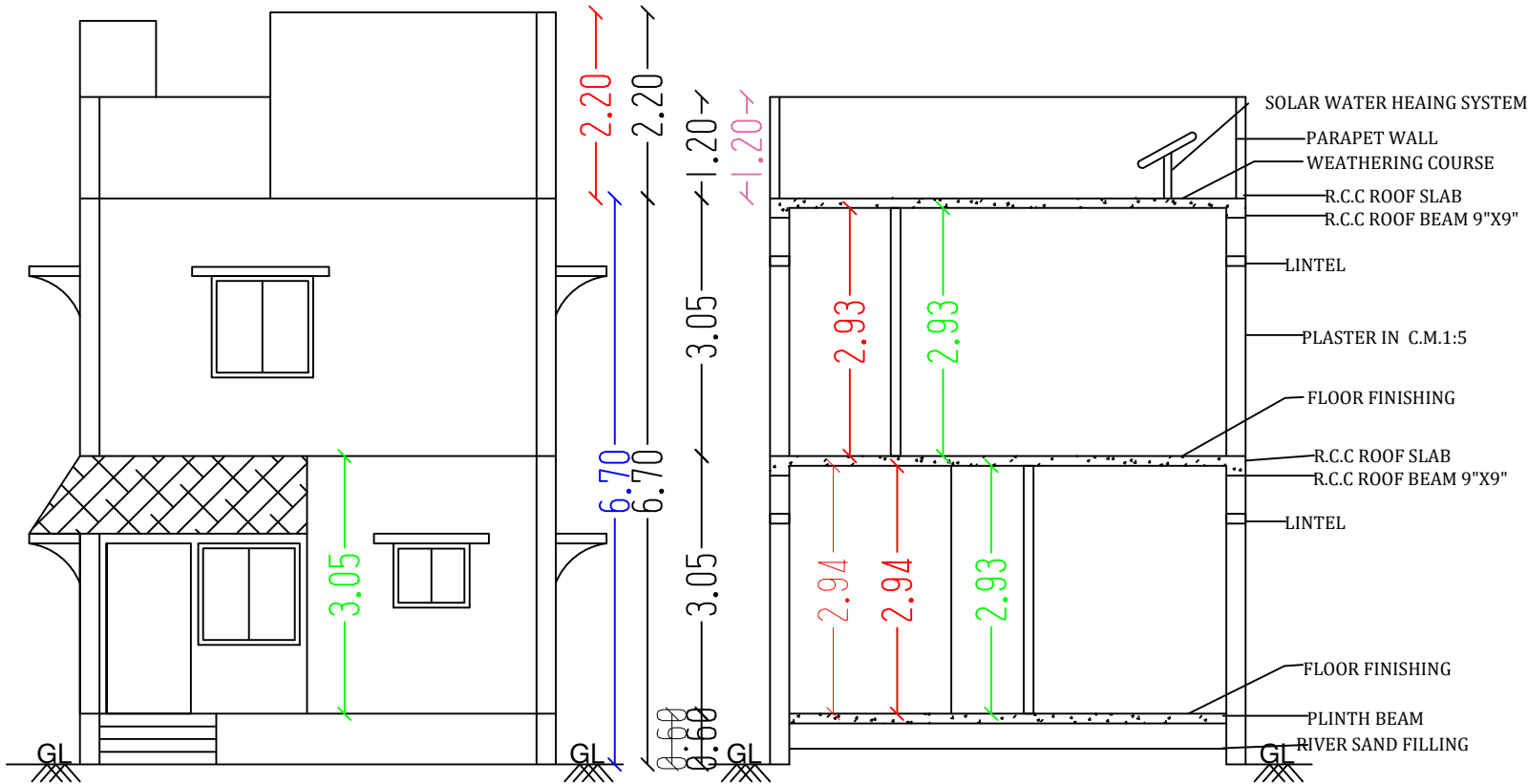
ELEVATION
