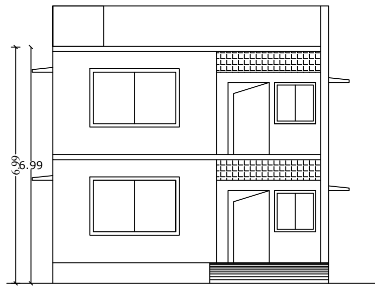
ELEVATION
