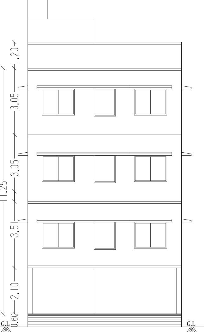
ELEVATION
