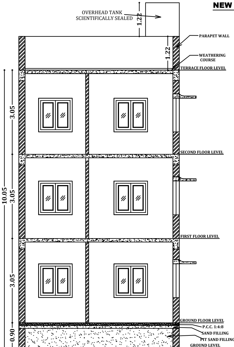
SECTION A-A'
