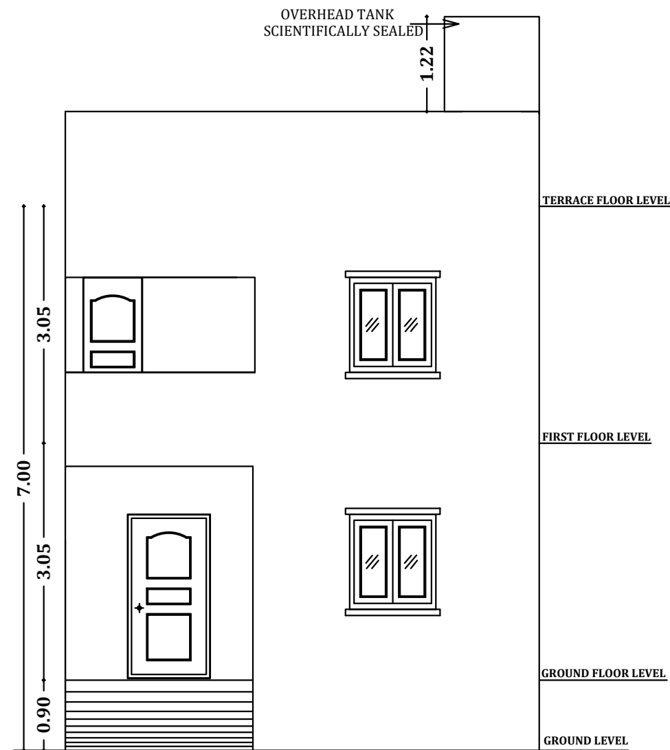
ELEVATION
