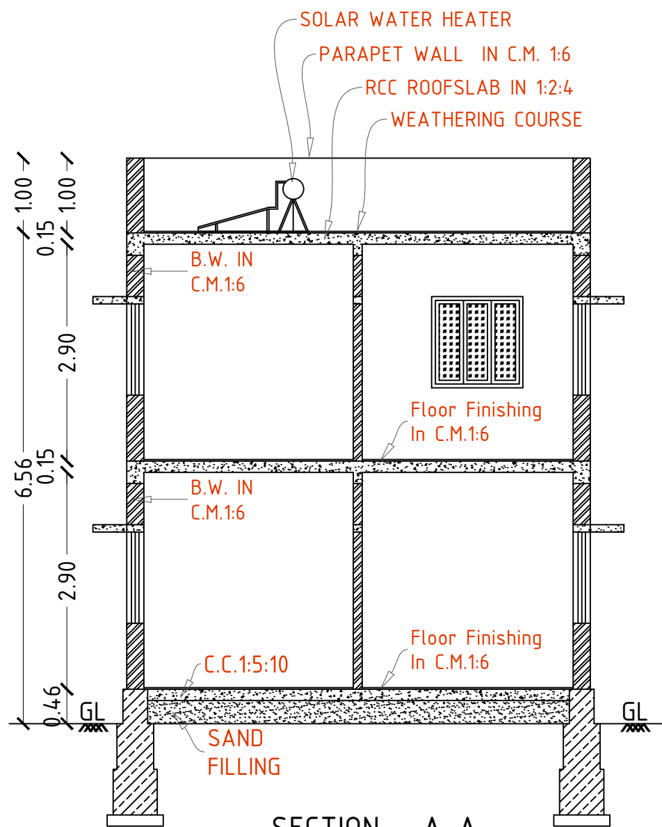
SECTION - A-A
