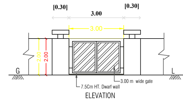
ELEVATION
