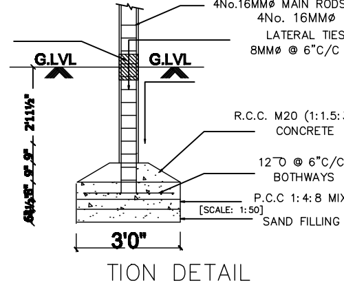
TION DETAIL
