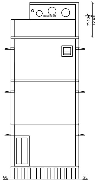
ELEVATION
