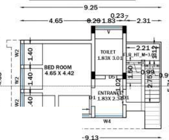
DOOR PLAN
