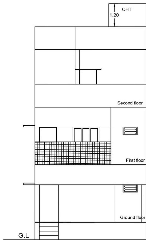
ELEVATION
