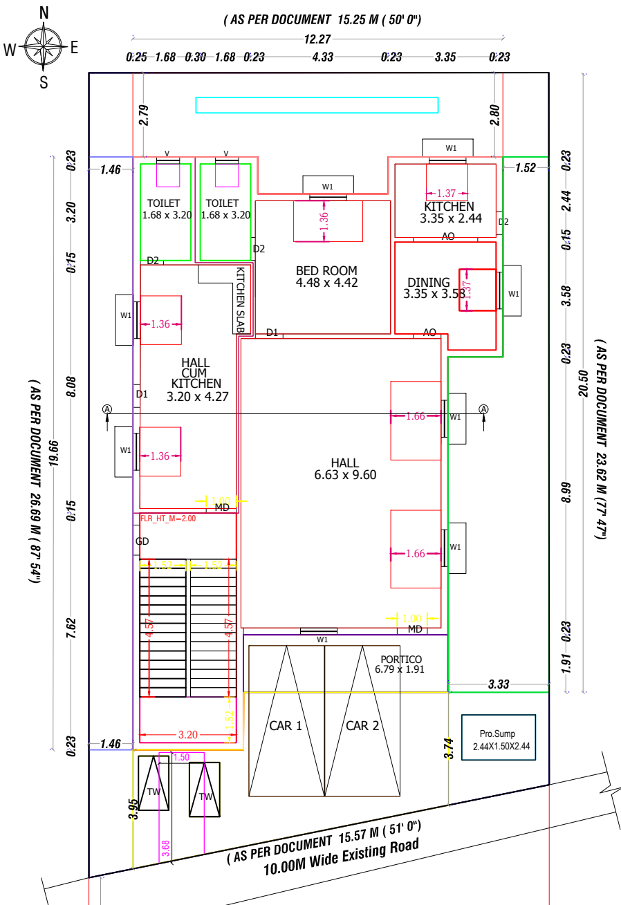
DOOR PLAN
