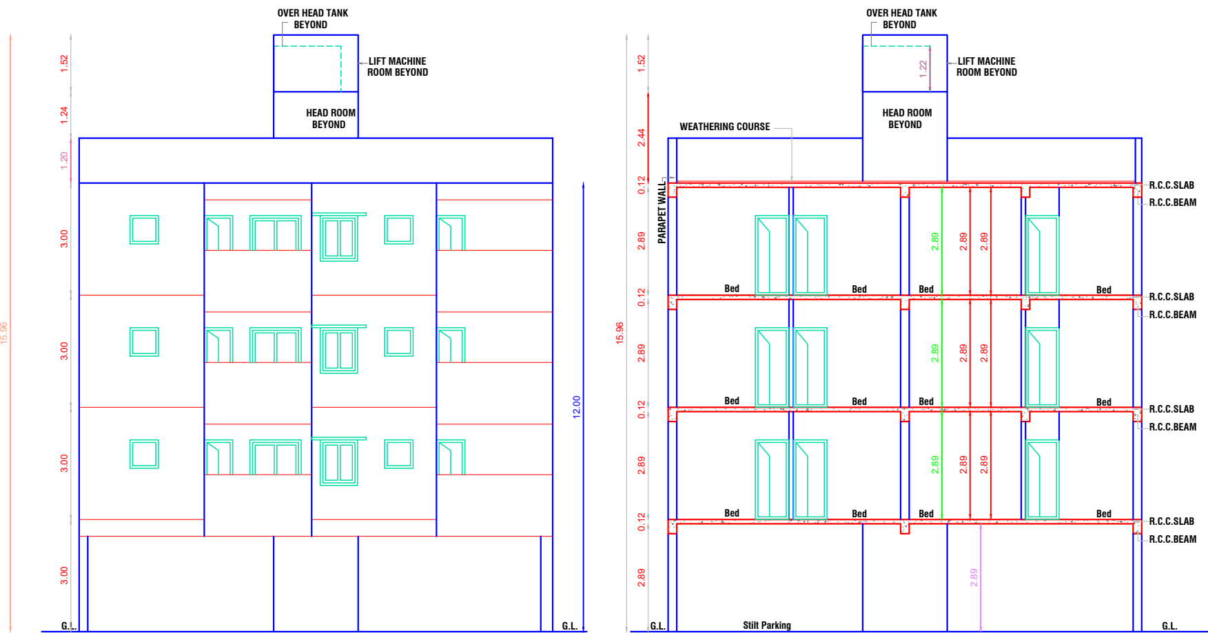
ELEVATION
