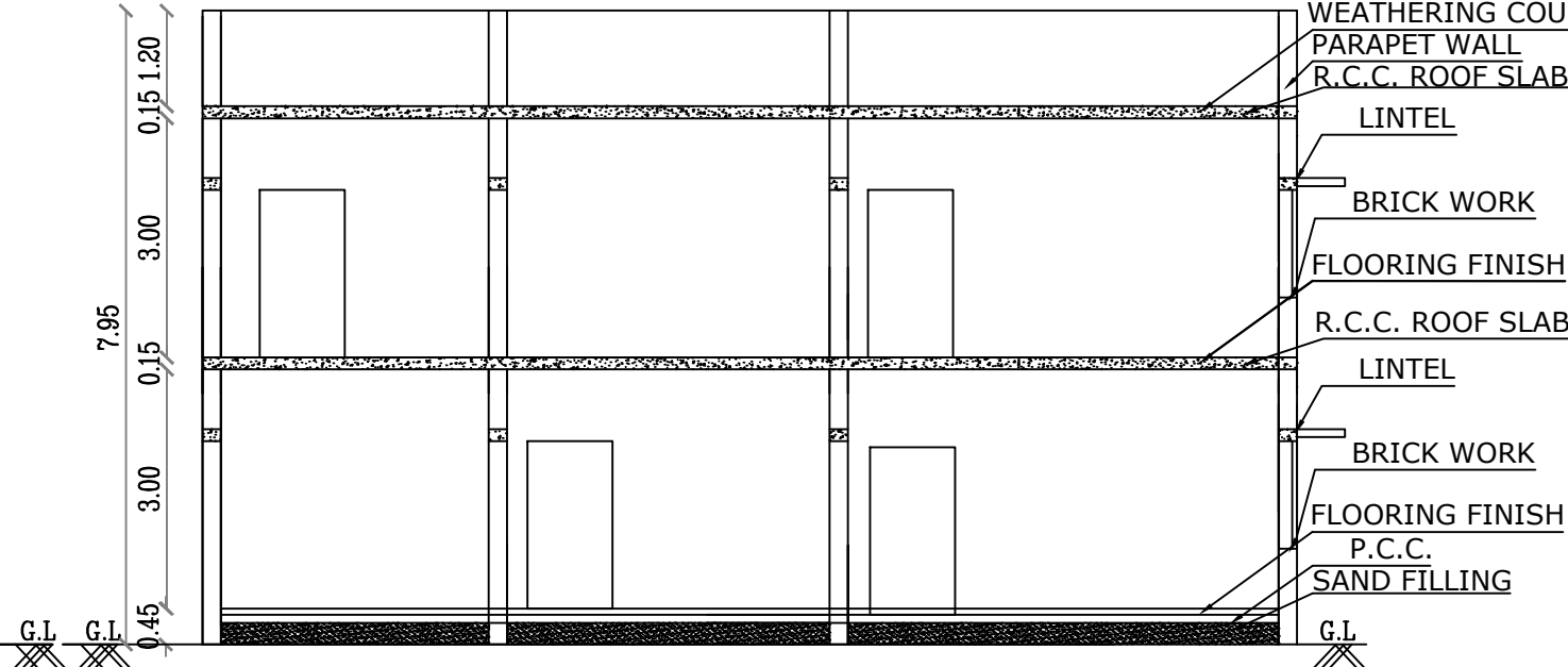
SECTION A-B
