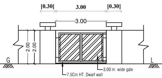
ELEVATION
