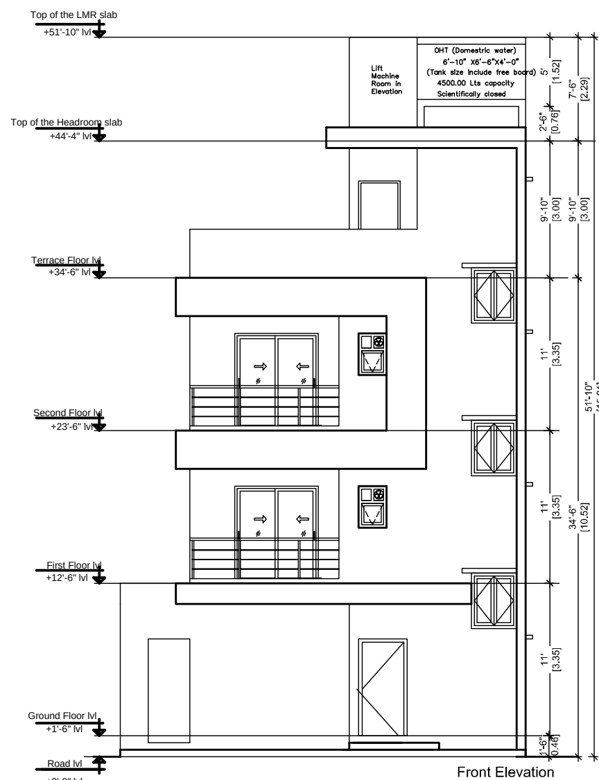
ELEVATION
