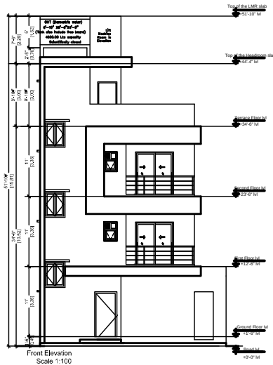
ELEVATION
