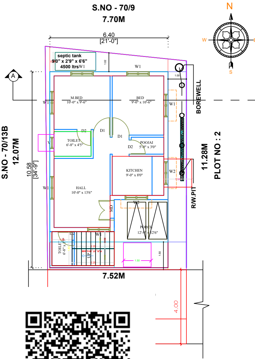
DOOR PLAN
