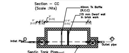
Section - CC (Scale : Nts)
