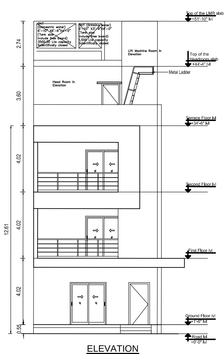
ELEVATION
