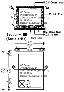
UG Sump Plan (Scale : Nts)
