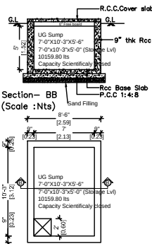
UG Sump Plan (Scale : Nts)
