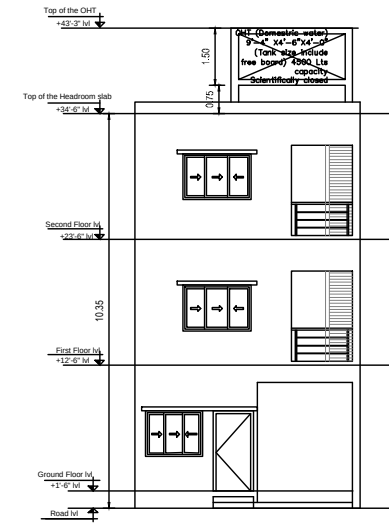
ELEVATION
