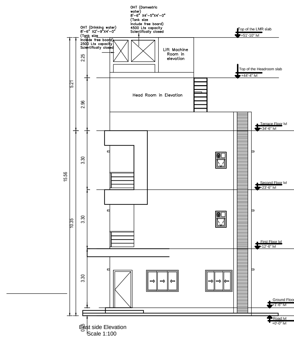
ELEVATION
