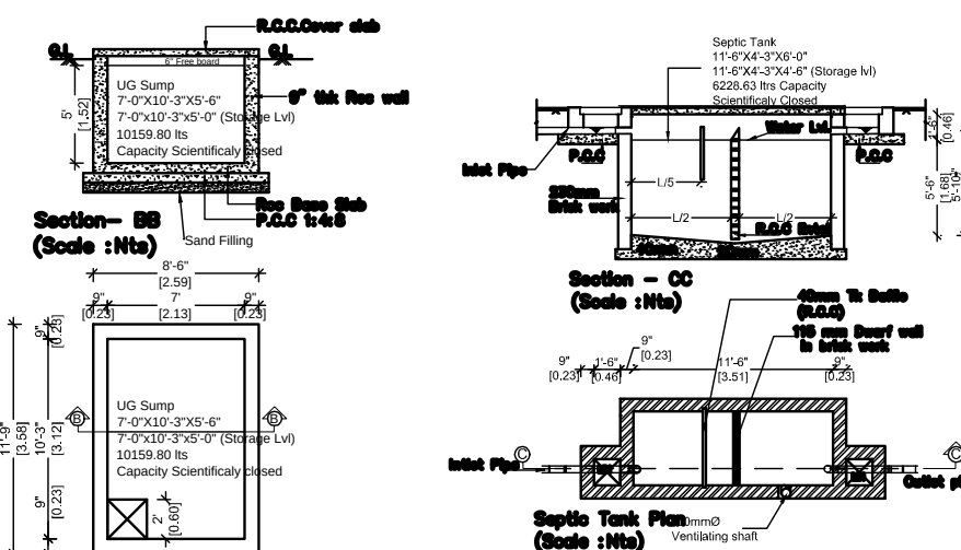
UG Sump Plan (Scale : Nts)
