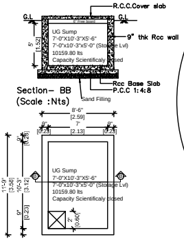
UG Sump Plan (Scale : Nts)
