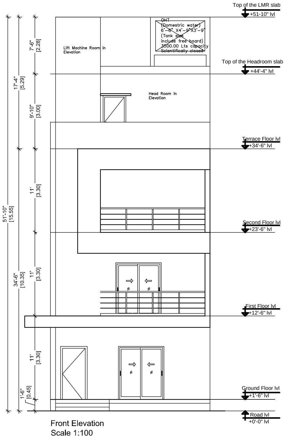
ELEVATION
