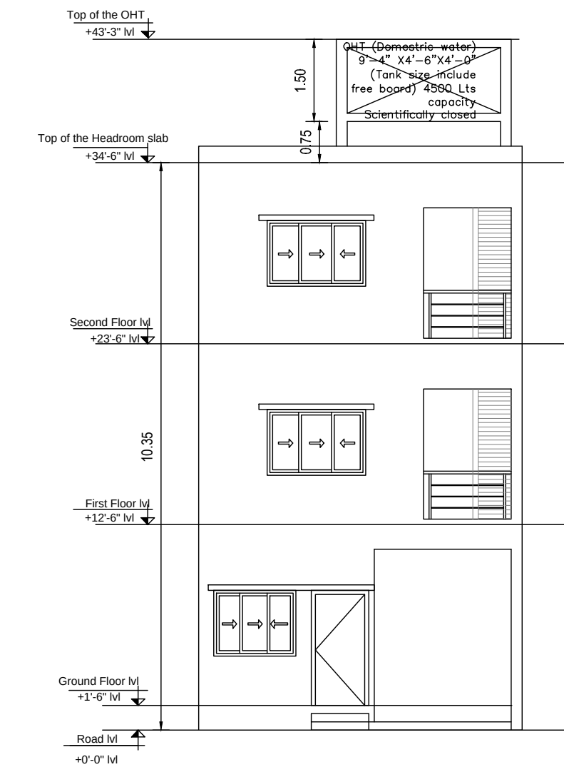
ELEVATION
