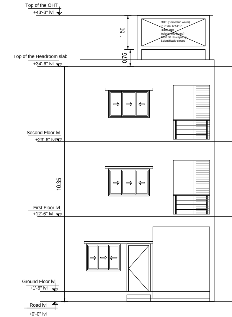
ELEVATION
