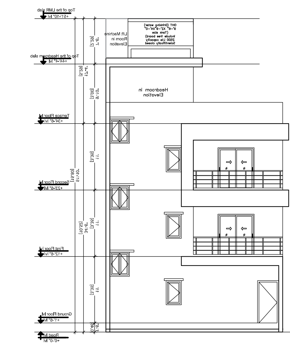
ELEVATION
