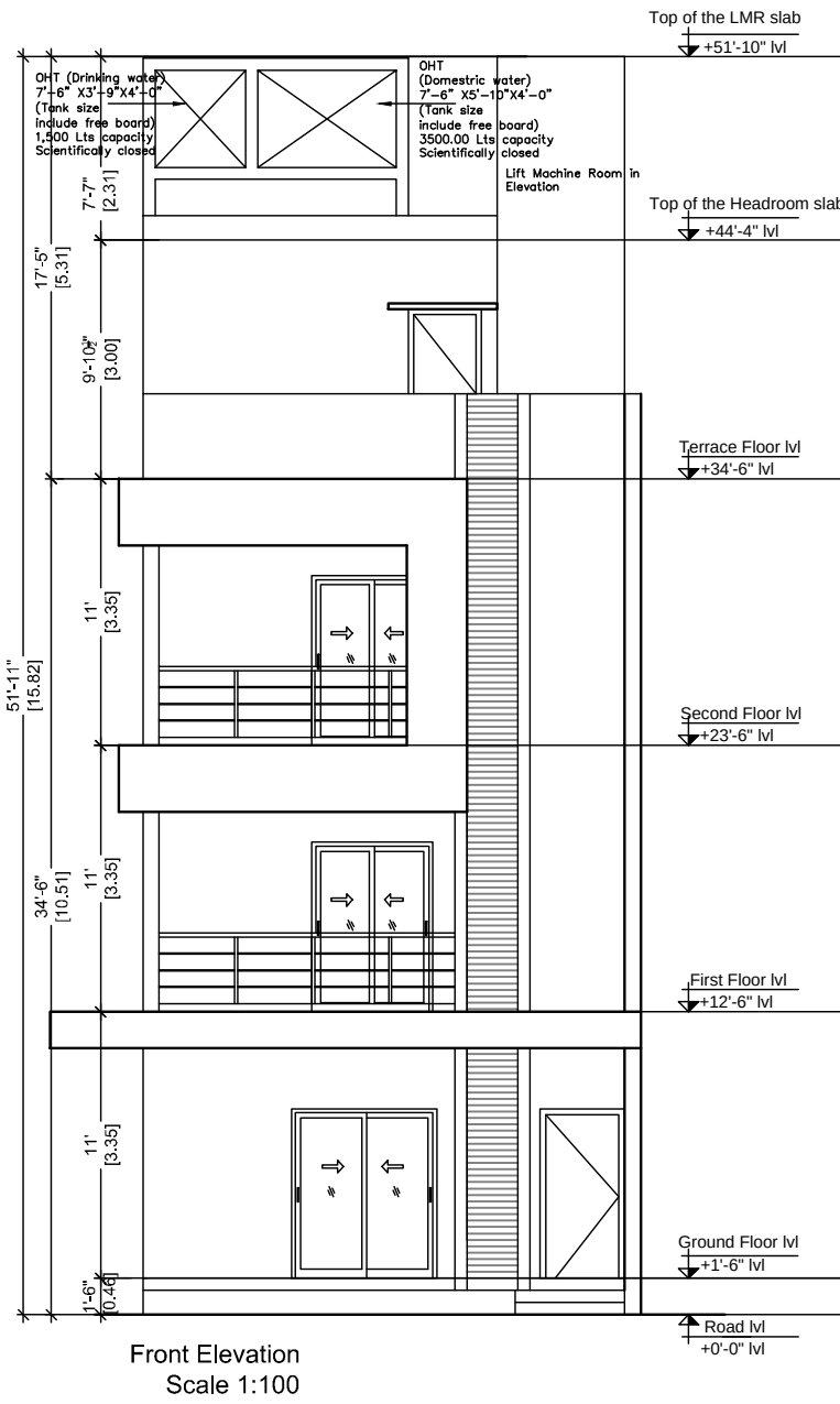
ELEVATION
