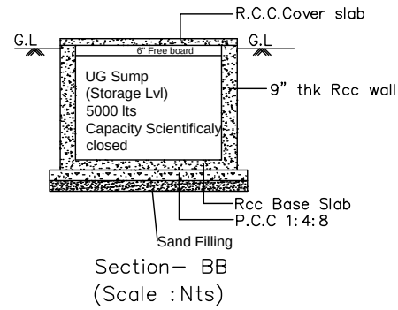
Section- BB (Scale : Nts)
