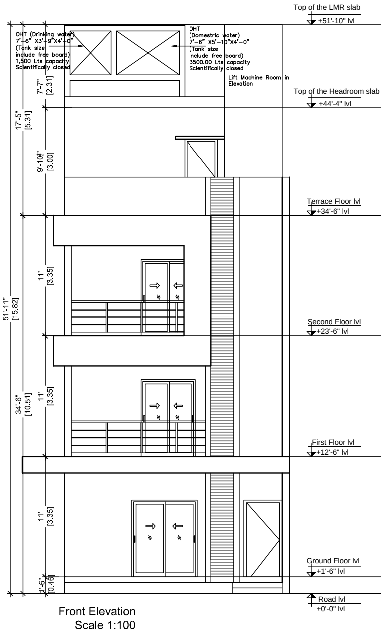
ELEVATION
