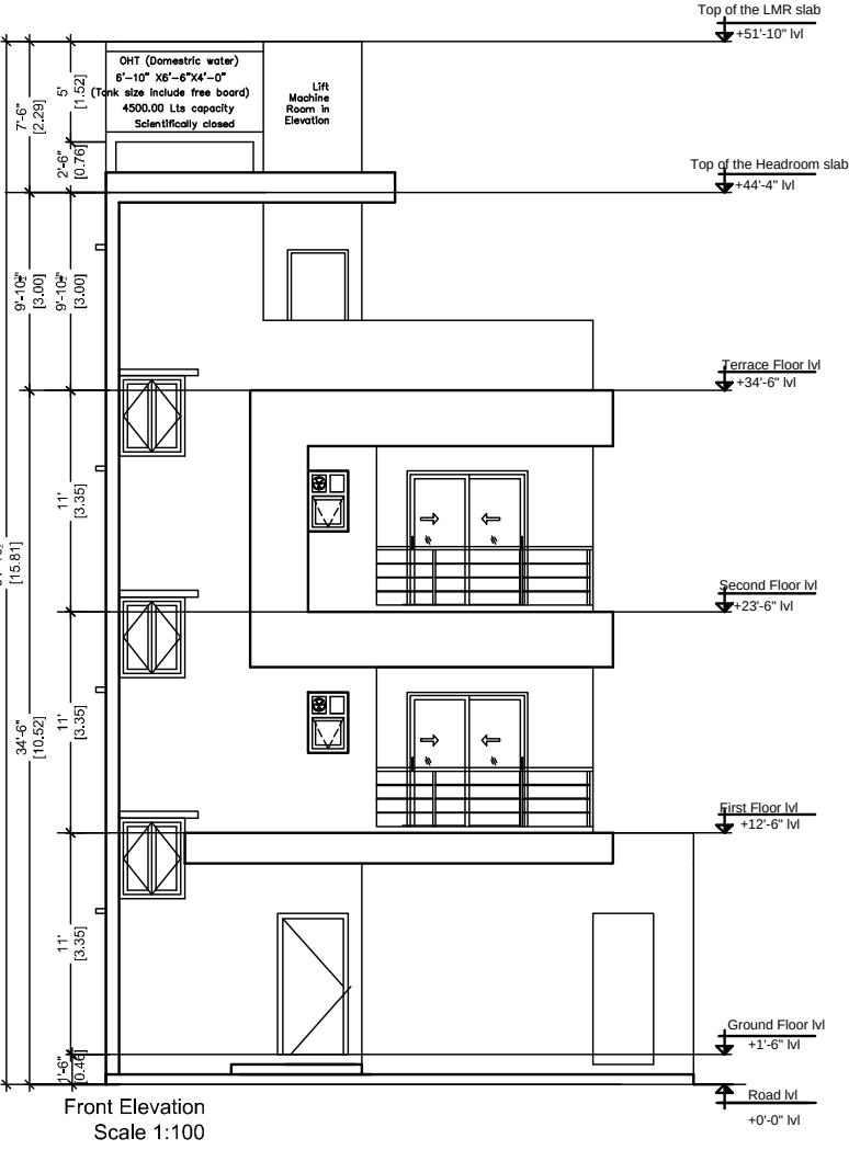
ELEVATION
