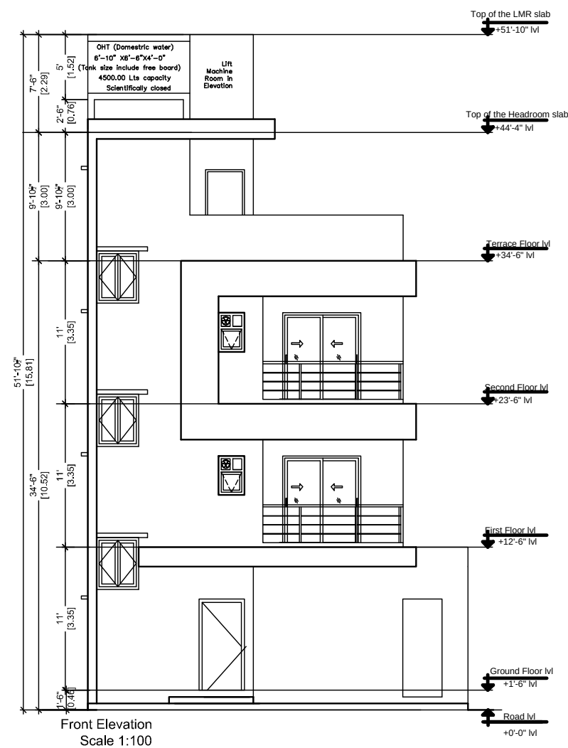
ELEVATION
