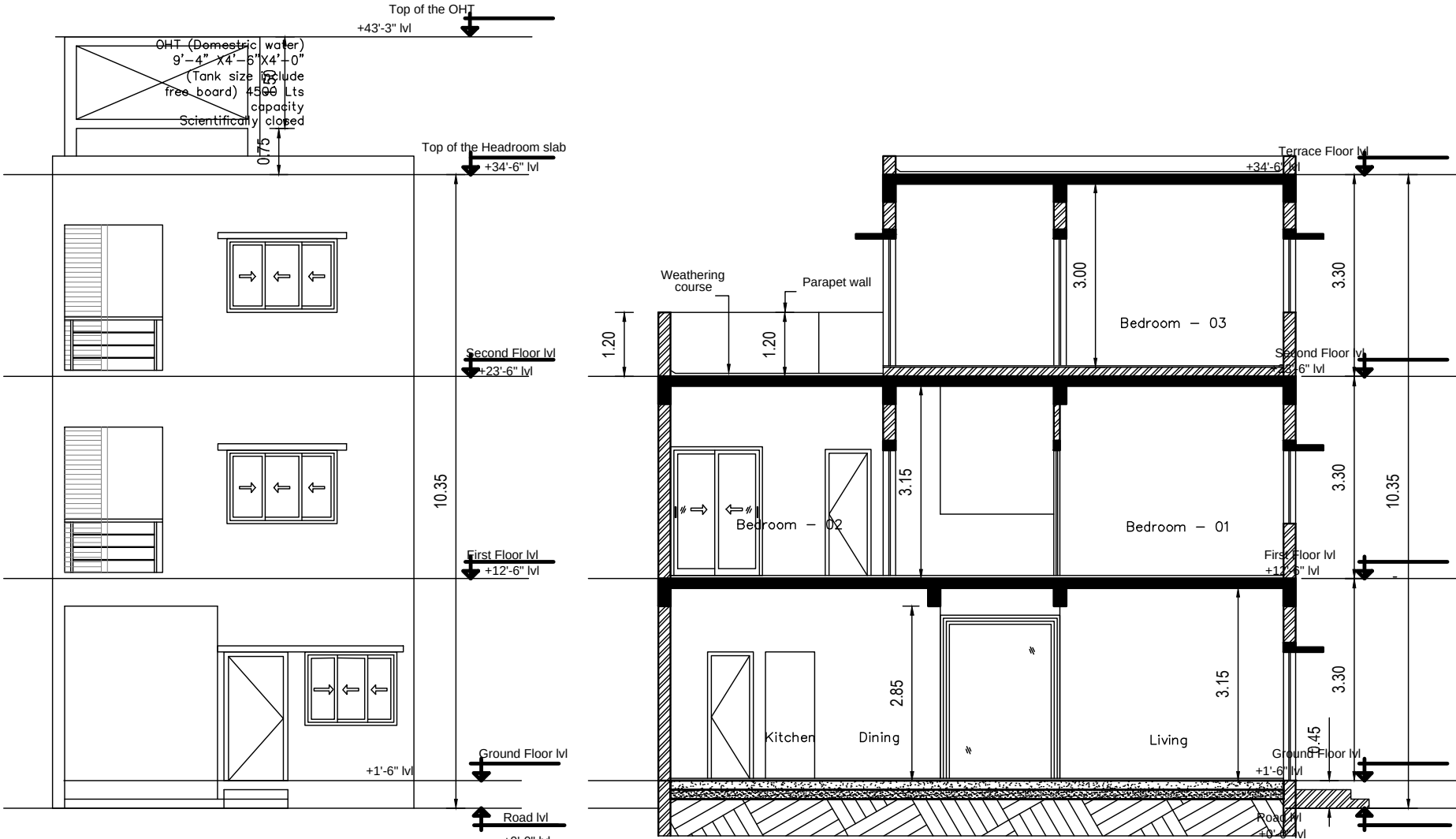
ELEVATION
