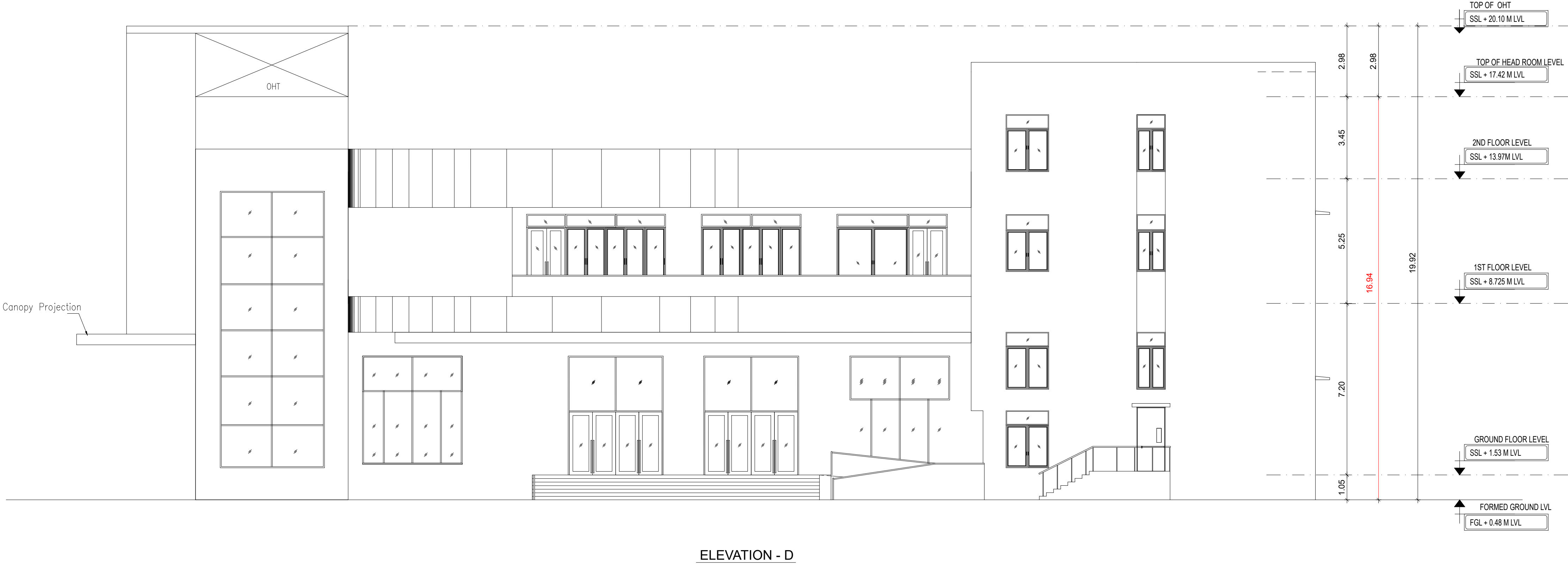
ELEVATION - D
