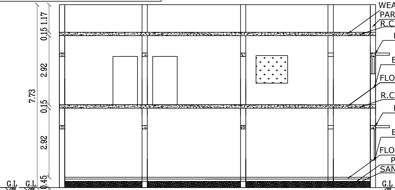
SECTION A-B
