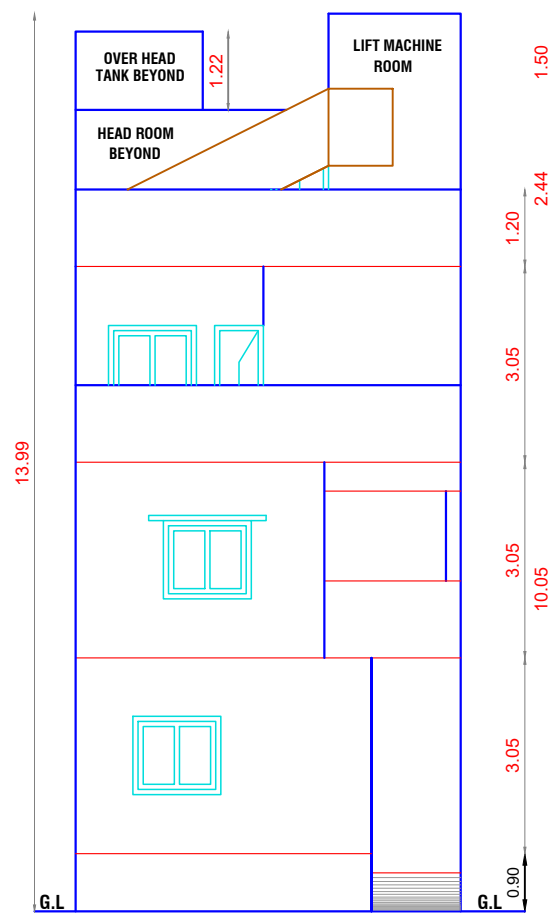
ELEVATION
