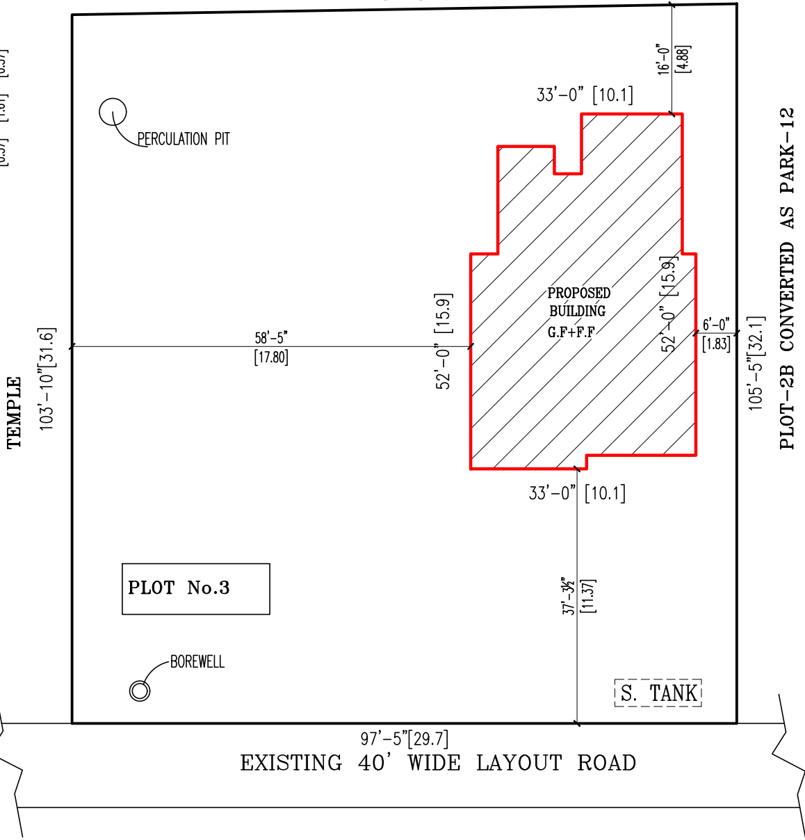
SITE PLAN(SCALE 1:200)
