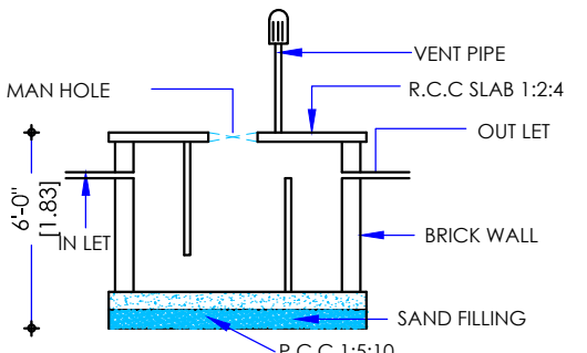
SECTION E,F
