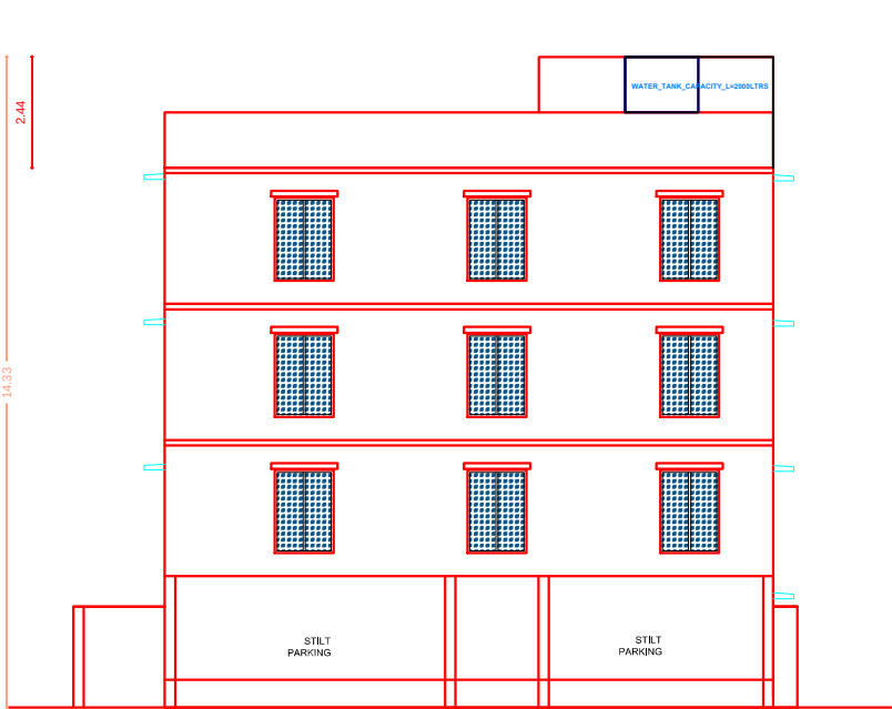
ELEVATION A
