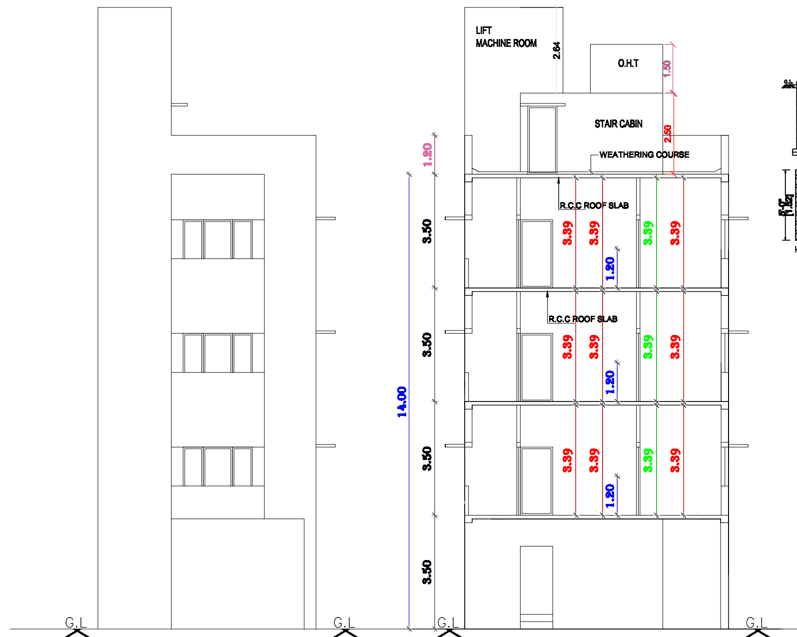
ELEVATION
