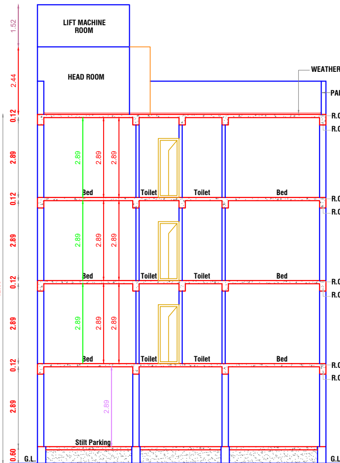
SECTION A-A
