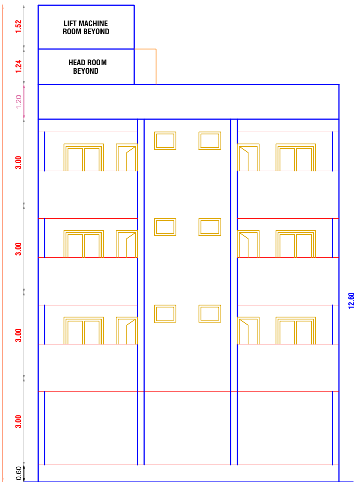
ELEVATION
