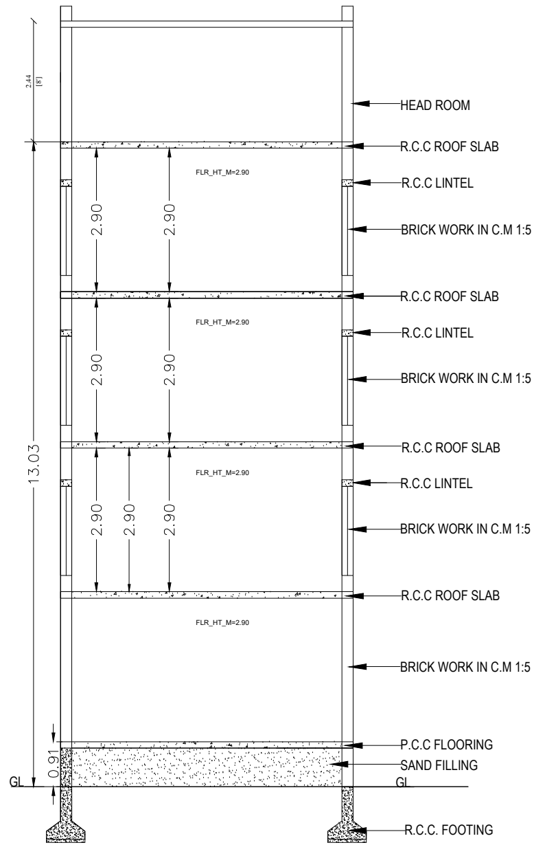
SECTION A-A
