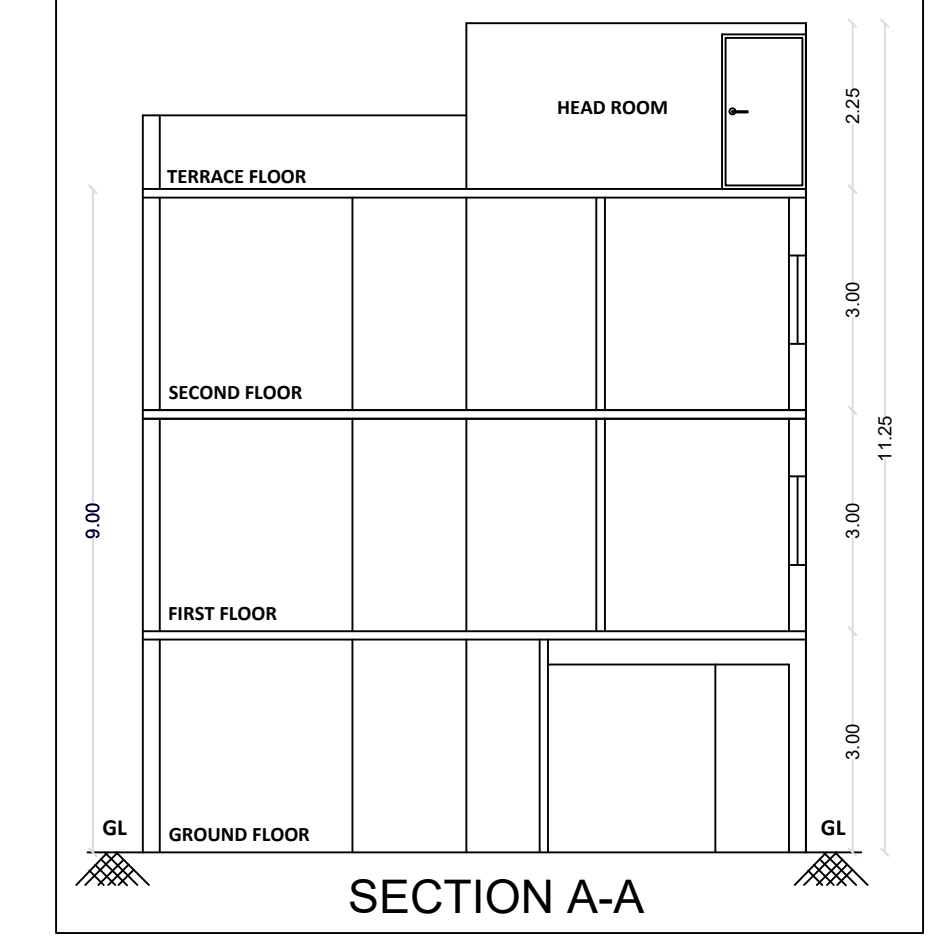
SECTION A-A
