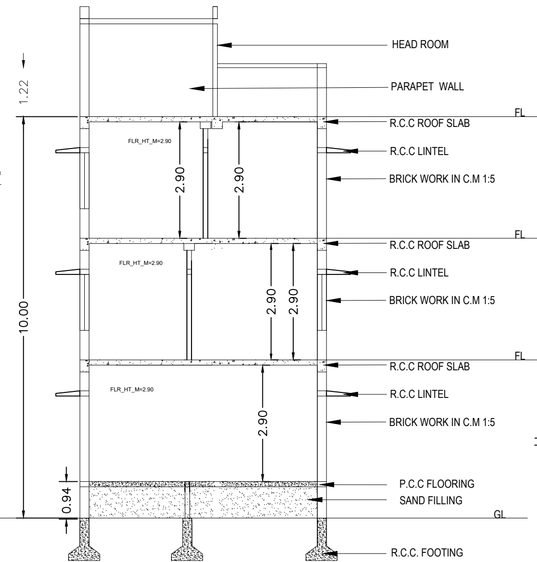
SECTION A-A
