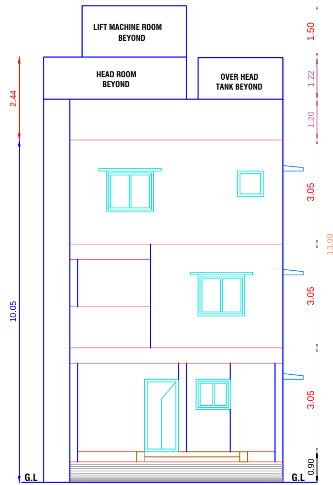
ELEVATION
