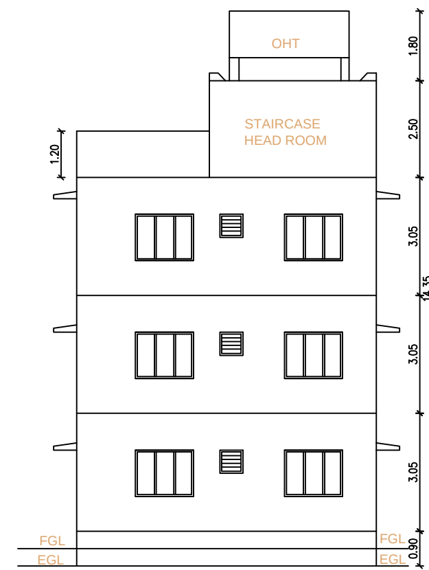
ELEVATION - A
