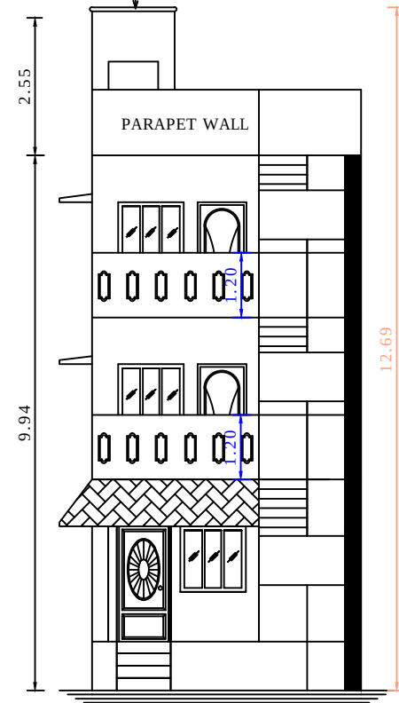
ELEVATION
