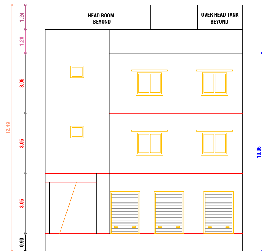
ELEVATION
