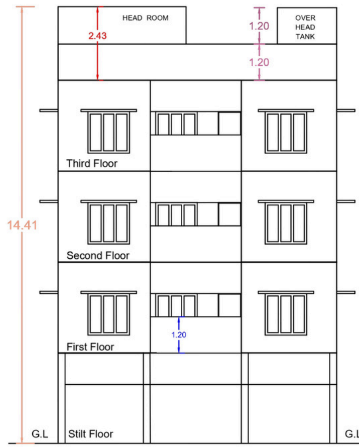
ELEVATION
