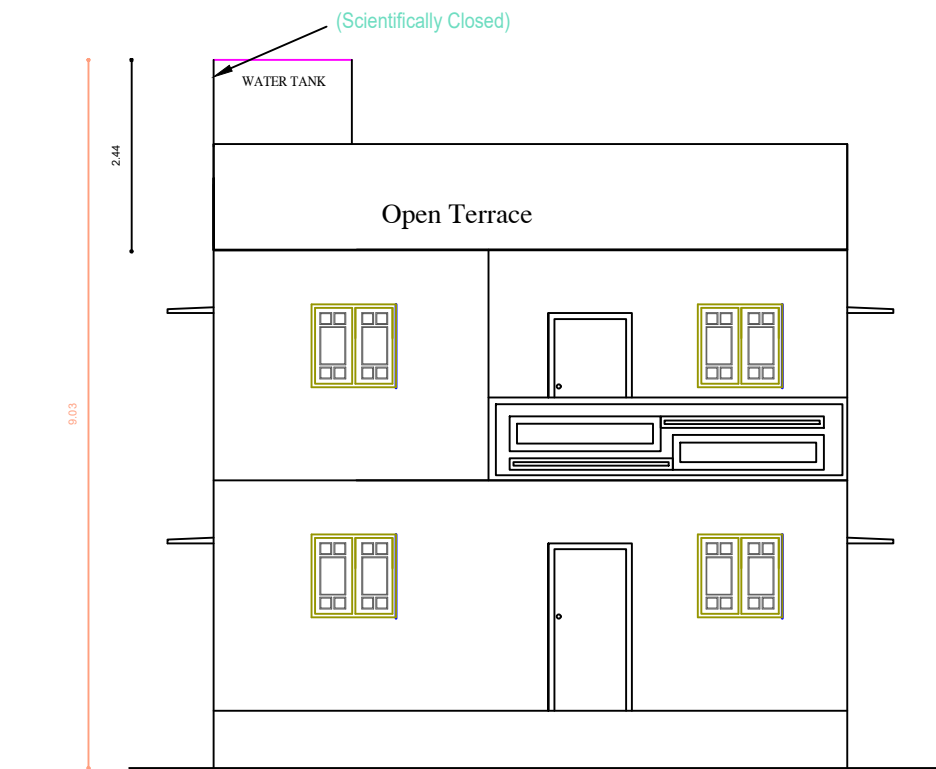
ELEVATION
